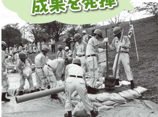
「月の輪工法」に取り組む水防団員
