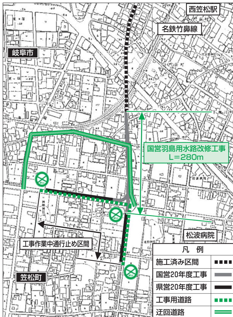
工事による交通規制予定図 (期間10月下旬～3月下旬)
