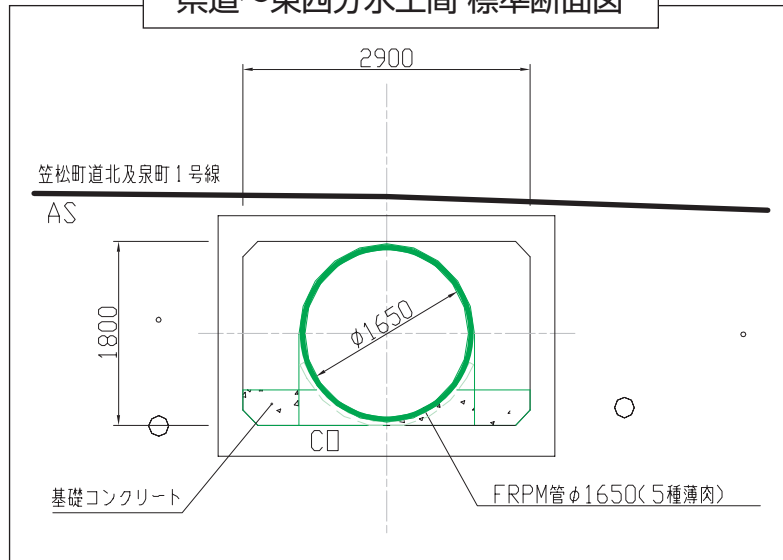
県道～東西分水工間 標準断面図
